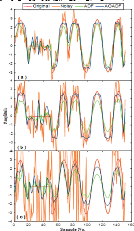
شکل ۴: ردیف ۱۷۵ داده‌های اصلی بدون نوفه، حاوی نوفه و خروجی فیلتر شده در شکل ۲-۲ در حالتی که داده اصلی با نوفه گاوسی با واریانس یک (a)، دو (b) و چهار (c) جمع شده است.
