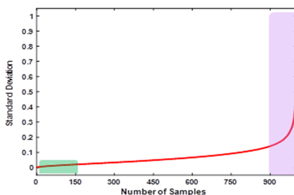
شکل ۳: میزان انحراف معیار محاسبه شده برای خروجی ۱۵ فیلتر ADF محاسبه شده برای پنج درصد از داده‌های شکل ۲b. مستطیل سبز، نشانگر نقاطی است که بیشترین احتمال تعلق به فضای رویدادهای همدوس را داشته‌اند و مستطیل بنفش، متناظر با نقاطی است که احتمال تعلق آنها به فضای رویدادهای تصادفی بیشتر است.
