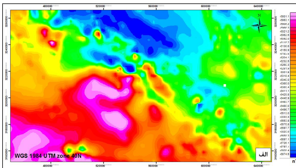
شکل ۲: نقشه‌های شبکه‌بندی تهیه شده با استفاده از نرم‌افزار Oasis montaj. (الف) نقشه میدان مغناطیسی پس از تصحیح IGRF. (ب) نقشه میدان مغناطیسی پس از اعمال فیلتر RTP. (ج) نقشه میدان مغناطیسی پس از اعمال فیلتر میان‌گذر.
