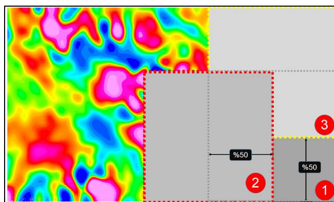
شکل ۳: نمونه‌ای از بلوک‌بندی با ابعاد ۸۰×۸۰ کیلومتر و هم‌پوشانی ۵۰٪.
