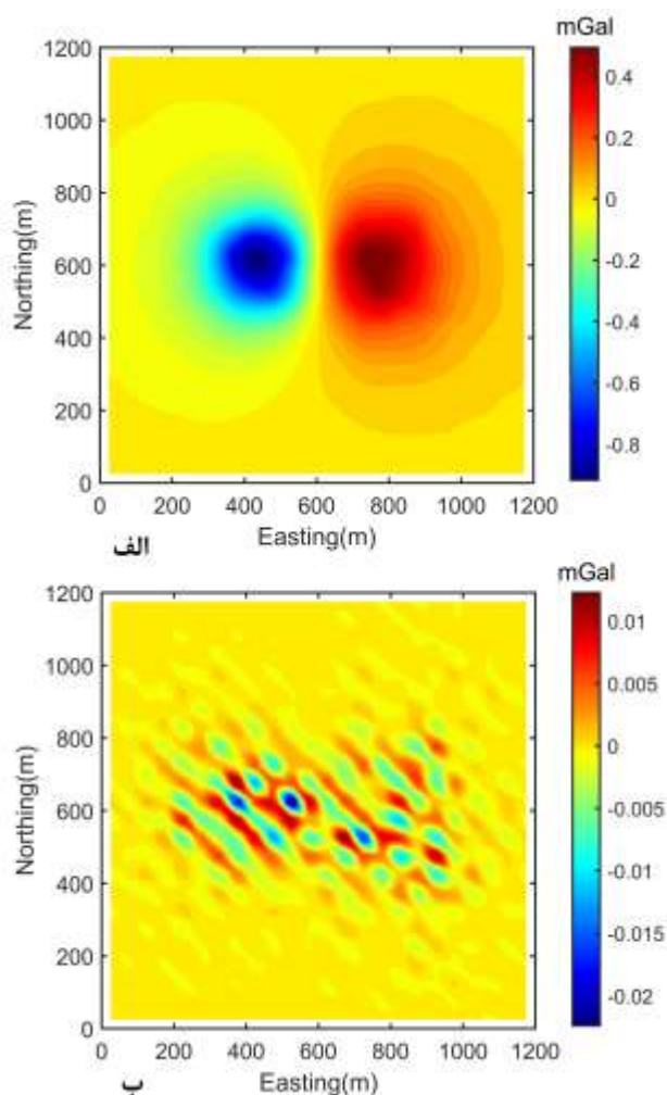
شکل ۳: داده‌های حاصل از مدل وارون (الف) نقشه اختلاف بین داده‌های
