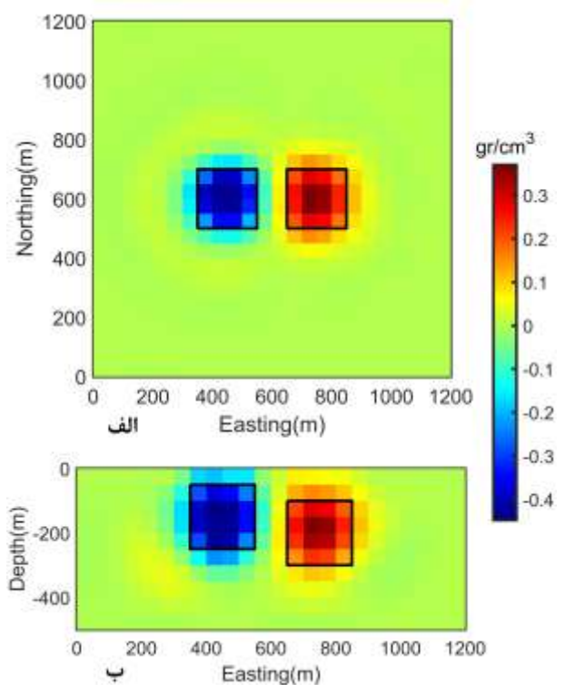
شکل ۴: مقطع افقی در مدل وارون در عمق ۱۵۰ متری از سطح زمین
