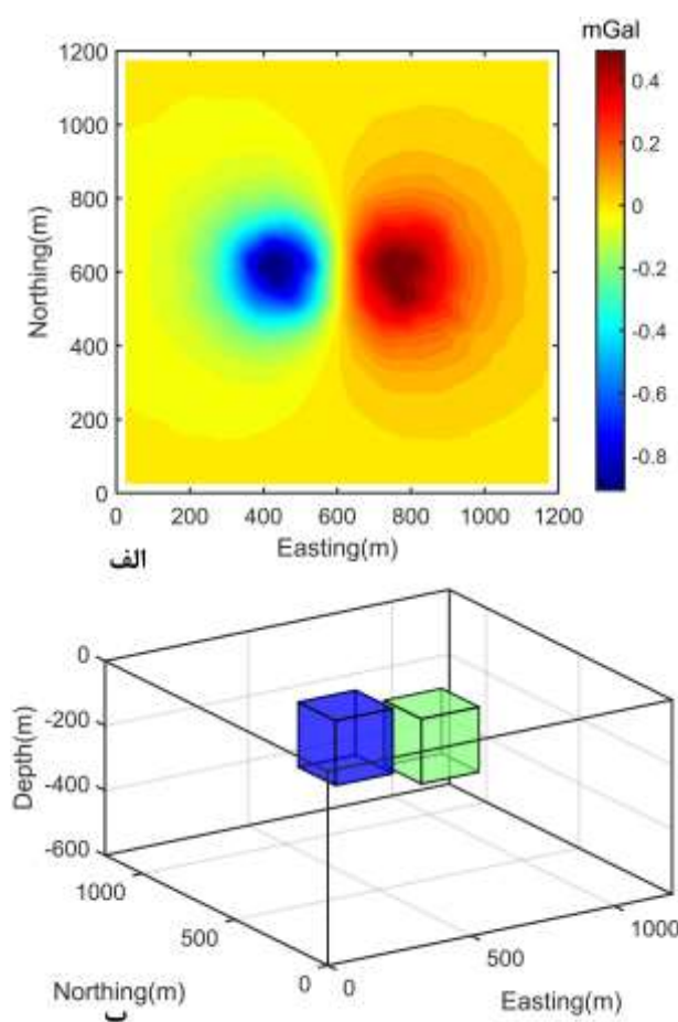
شکل ۲: داده‌های حاصل از مدل مصنوعی (الف). نمای سه بعدی مدل
