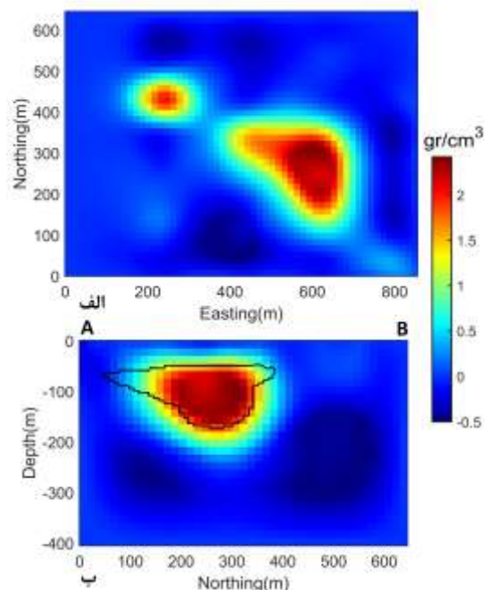
شکل ۱۰: مقطع افقی در عمق ۷۵ متری (الف) و مقطع قائم در امتداد A-
