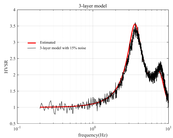
شکل ۸: تخمین HVSr مدل B با ۱۵٪ نوفه توسط الگوریتم CJaya (نمودار مشکی رنگ بیانگر مدل مشاهده شده همراه با نوفه و نمودار قرمز رنگ خروجی CJaya)
