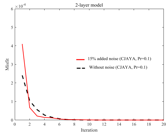
شکل ۳: مقایسه نرخ همگرایی الگوریتم CJaya در وارون‌سازی مدل A با نوفه و بدون آن
