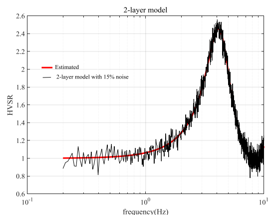
شکل ۴: تخمین HVSR مدل A با ۱۵٪ نوفه توسط الگوریتم CJaya (نمودار مشکی رنگ بیانگر مدل مشاهده شده همراه با نوفه و نمودار قرمز رنگ خروجی CJaya )
