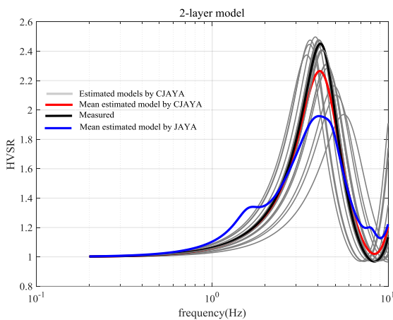
شکل ۲: مقایسه الگوریتم‌ها در تخمین HVSr مدل A (نمودار مشکی رنگ بیانگر مدل مشاهده شده، نمودار آبی رنگ خروجی Jaya و نمودار قرمز رنگ خروجی CJaya)
