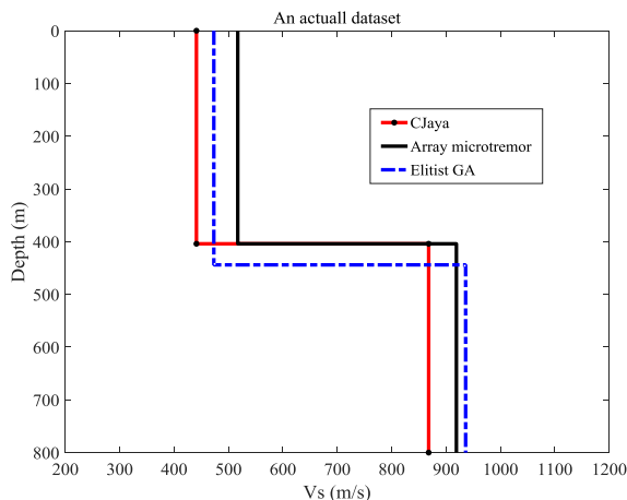
شکل ۱۲: مدلسازی Vs در ایستگاه مورد مطالعه با استفاده از CJaya (نمودار قرمز)، Elitist GA (نمودار منقطع آبی رنگ) و مایکروترمور (نمودار مشکی رنگ)
