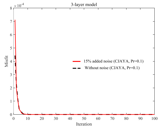
شکل ۷: مقایسه نرخ همگرایی الگوریتم CJaya در وارون‌سازی مدل B با نوفه و بدون آن
