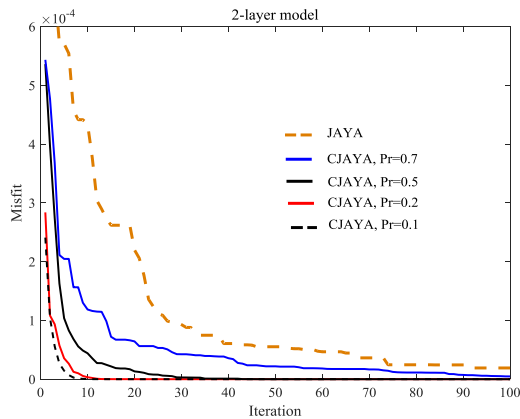
شکل ۱: مقایسه نرخ همگرایی الگوریتم CJaya و Jaya در وارون‌سازی مدل A
