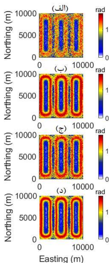
شکل ۵: محاسبه زاویه تیلت افقی برای داده‌های گرانی مصنوعی با ۳ درصد نوفه گاوسی با استفاده از روش: (الف) دامنه فرکانسی، (ب) تفاضل پسرو، (ج) بسط تیلور-ادامه فراسو، (د) تفاضل محدود-ادامه فراسو
