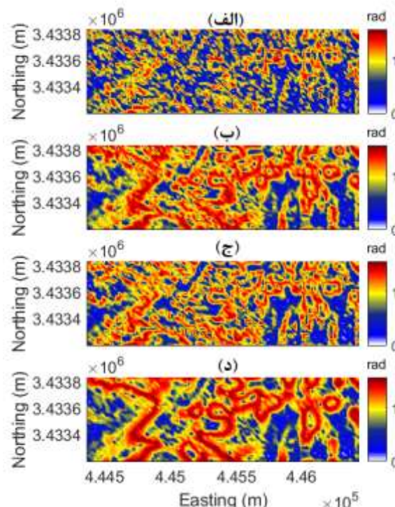
شکل ۱۴: محاسبه زاویه تیلت افقی برای داده‌های گرانی واقعی با استفاده از روش: (الف) دامنه فرکانسی، (ب) تفاضل پسر، (ج) بسط تیلور-ادامه فراسو، (د) تفاضل محدود-ادامه فراسو
