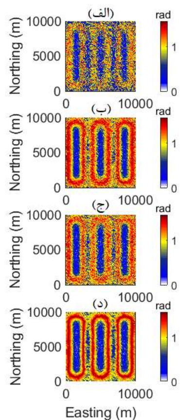
شکل ۶: محاسبه زاویه تیلت افقی برای داده‌های گرانی مصنوعی با ۳ درصد نوفه گاوسی با استفاده از روش: (الف) دامنه فرکانسی، (ب) تفاضل پسرو، (ج) بسط تیلور-ادامه فراسو، (د) تفاضل محدود-ادامه فراسو
