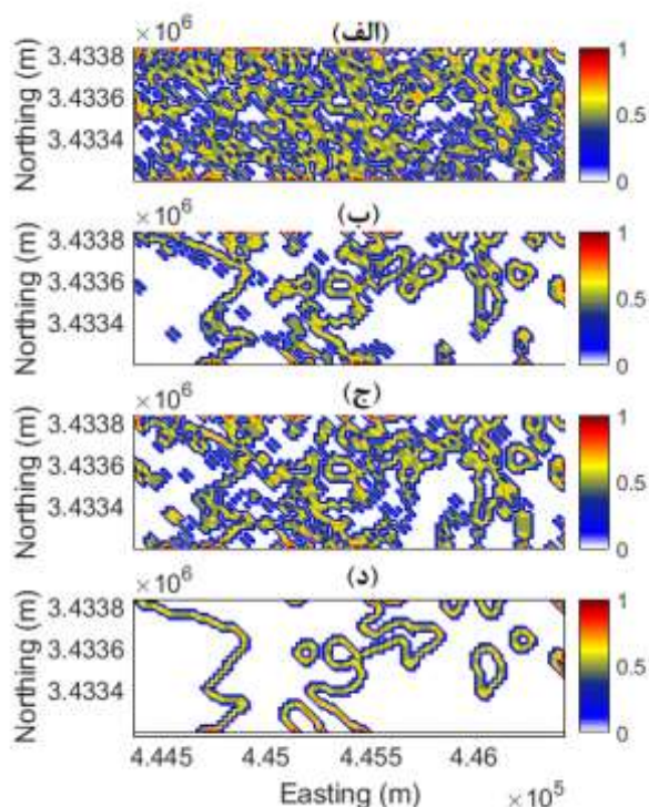
شکل ۱۳: تعیین مرز افقی با روش تابع هوی‌ساید برای داده‌های گرانی میدانی با استفاده از روش: (الف) دامنه فرکانسی، (ب) تفاضل پسر، (ج) بسط تیلور-ادامه فراسو، (د) تفاضل محدود-ادامه فراسو
