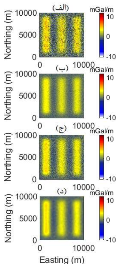
شکل ۴: محاسبه مشتق قائم داده‌های گرانی مصنوعی با ۶ درصد نوفه گاوسی با روش: (الف) دامنه فرکانسی، (ب) تفاضل پسرو، (ج) بسط تیلور-ادامه فراسو، (د) تفاضل محدود-ادامه فراسو
