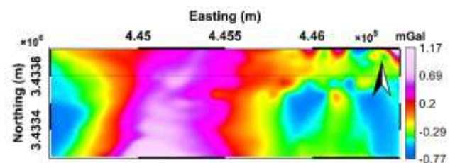
شکل ۱۰: نقشه بی‌هنجاری گرانی باقی‌مانده معدن جلال آباد بر حسب میلی‌گال
