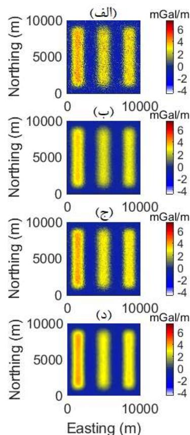
شکل ۳: محاسبه مشتق قائم داده‌های گرانی مصنوعی با ۳ درصد نوفه گاوسی با روش: (الف) دامنه فرکانسی، (ب) تفاضل پسرو، (ج) بسط تیلور-ادامه فراسو، (د) تفاضل محدود-ادامه فراسو
