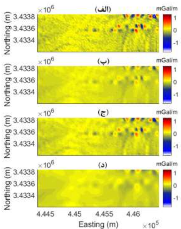
شکل ۱۱: محاسبه مشتق قائم داده‌های گرانی محدوده مورد مطالعه با روش: (الف) دامنه فرکانسی، (ب) تفاضل پسر، (ج) بسط تیلور-ادامه فراسو، (د) تفاضل محدوده-ادامه فراسو
