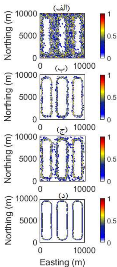
شکل ۷: تعیین مرز افقی با فیلتر تابع هوی‌ساید برای داده‌های گرانی مصنوعی با ۳ درصد نوفه گاوسی با استفاده از روش: (الف) دامنه فرکانسی، (ب) تفاضل پسرو، (ج) بسط تیلور-ادامه فراسو، (د) تفاضل محدود-ادامه فراسو
