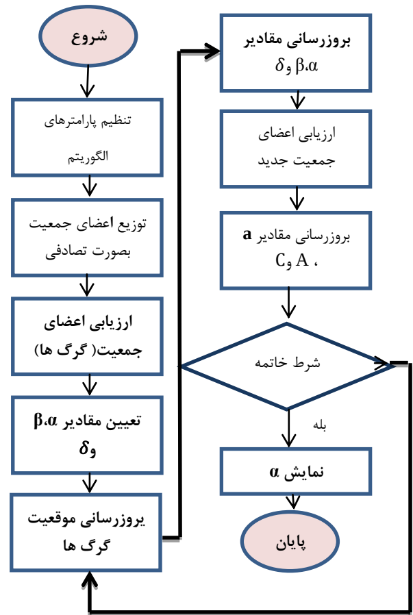
شکل ۵: فلوچارت الگوریتم GWO
