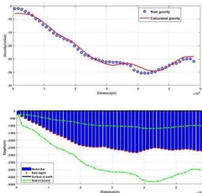
شکل ۱۱. مدلسازی دوبعدی پروفیل گرانی حوضه رسوبی مغان: بیهنجاری گرانی محاسبه شده و داده های برداشت شده (تصویر بالا)، مدل تولید شده (تصویر پایین)
