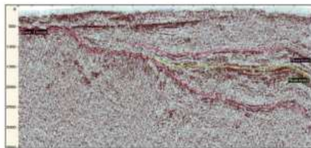
شکل ۱۳. مدل سازی پیشتر انجام شده مقطع مورد مطالعه به وسیله الگوریتم رقابت ذرات (جولایی و همکاران، ۱۳۹۸).
