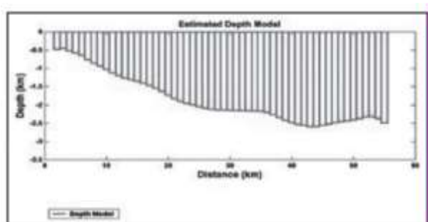
شکل ۱۲. مدل سازی پیشتر انجام شده مقطع مورد مطالعه به وسیله الگوریتم مارکورات -لونبرگ (نجاتی و همکاران، ۱۳۸۸).
