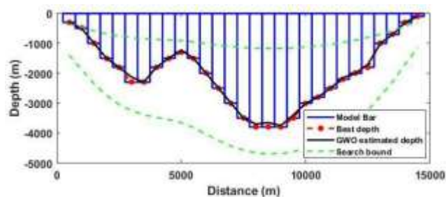
شکل ۷: الف) داده‌های مصنوعی به همراه داده‌های مدل تولیدی (تصویر بالا)، مدل مصنوعی به همراه مدل تولیدی (تصویر پایین)
