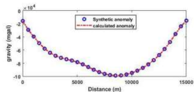
شکل ۶: مدل مصنوعی دو بعدی یک حوضه رسوبی منشور بندی شده (تصویر پایین)، بیهنجاری گرانی بدست آمده از مدل مصنوعی قرار گرفته در بالای هر منشور (تصویر بالا)
