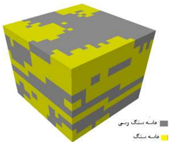
شکل ۱۴: نمونه‌ای از مدل‌های رخساره‌ای حاصل از اعمال روش روند احتمالی عمودی بر شبیه‌سازی شاخصی متوالی
