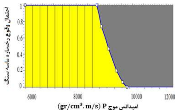
شکل ۱۳: تابع توزیع احتمال حضور رخساره‌ها نسبت به داده‌های امپدانس موج P به کار گرفته شده در روش روند احتمالی لرزه‌ای
