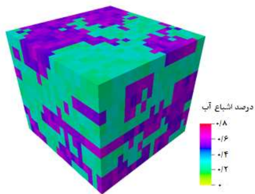
شکل ۴: مدل مرجع درصد اشباع آب متناظر با مدل رخساره‌ای مرجع
