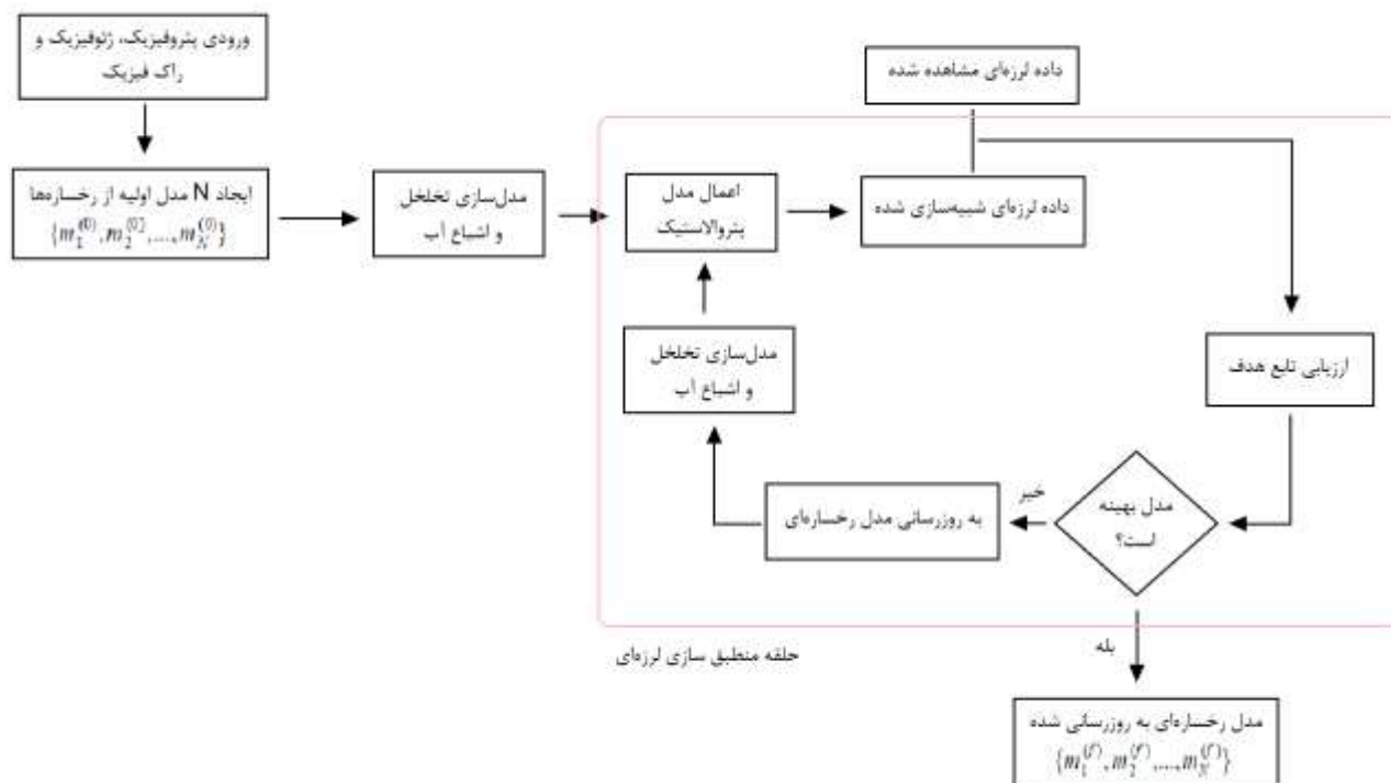
شکل ۱: مراحل اصلی روش چرخه انطباق با داده‌های لرزه‌ای
