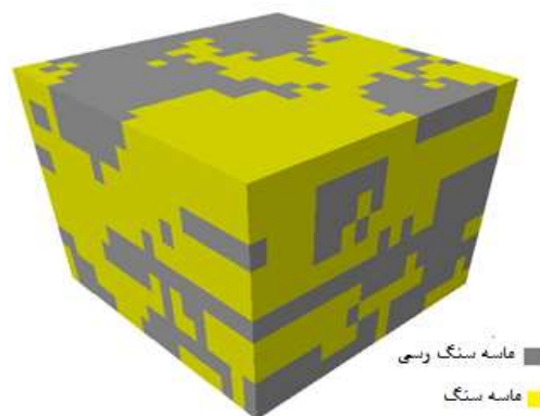
شکل ۱۰: یکی از مدل های رخساره ای به برورسانی شده بوسیله روش کلونی
