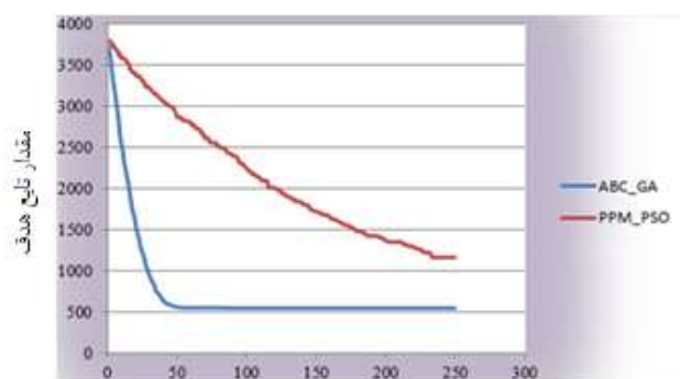
تکرار چرخه انطباق یا داده های لرزه ای
