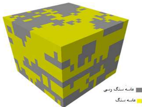
شکل ۸: یکی از مدل‌های رخساره‌ای بروزرسانی شده توسط روش آشفته‌گی احتمال - ازدحام ذرات
