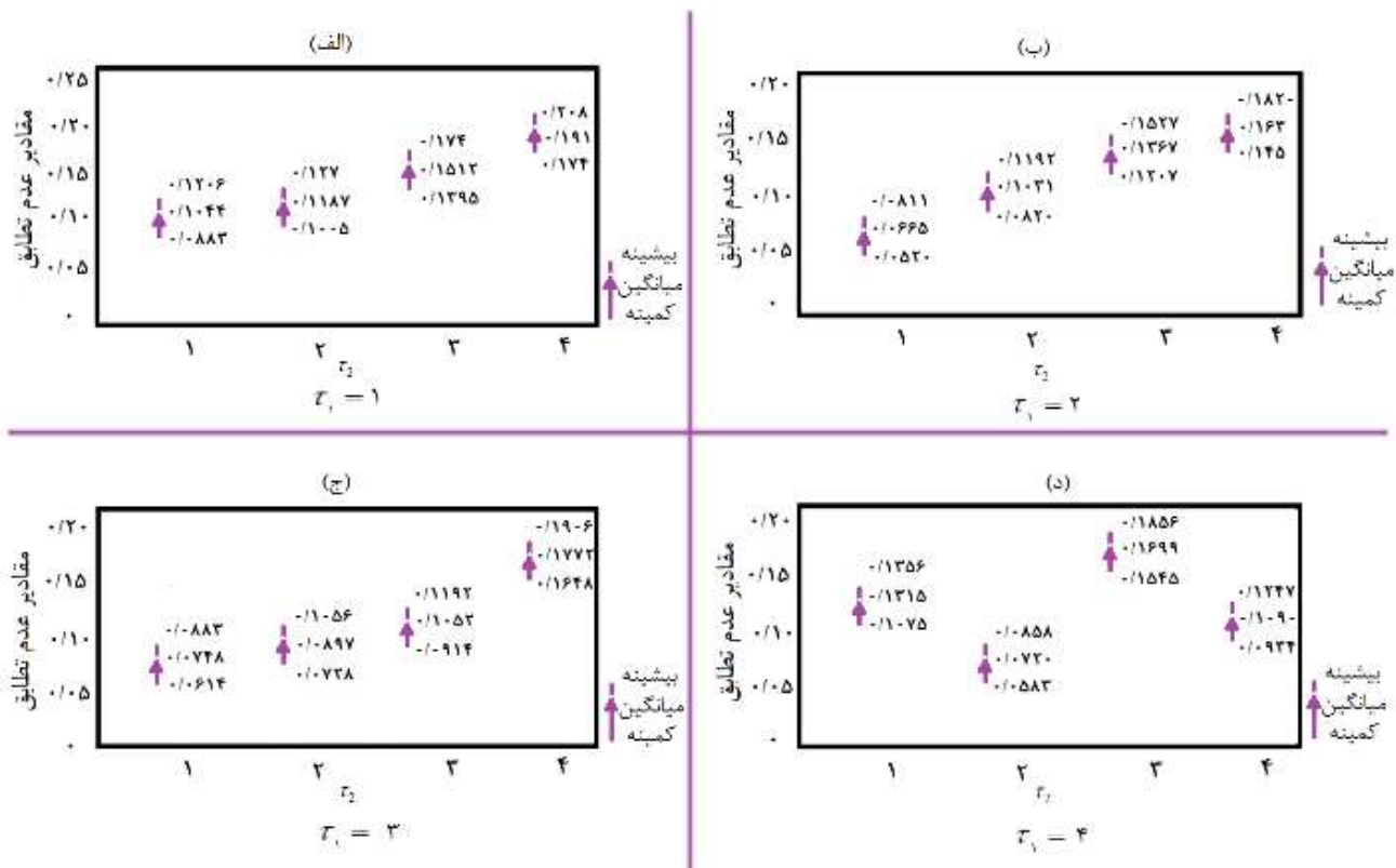
شکل ۹: آنالیز حساسیت پارامترهای ( T_1 ) و ( T_2 ) روش آشفته‌گی احتمال. این شکل نشان می‌دهد هنگامی که نسبت ( T_1 ) به ( T_2 ) برابر ۲ باشد، مقدار پارامتر عدم تطابق مدل‌های رخساره‌ای ساخته شده دارای مقادیر کمتری می‌باشد.
