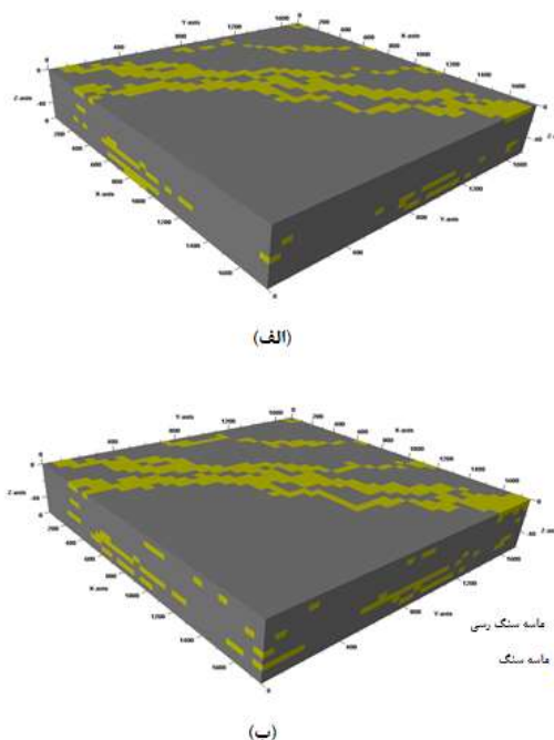
شکل ۱۸: الف) یک نمونه از مدل‌های رخساره‌ای کانالی بروز رسانی شده توسط روش کلونی زنبور مصنوعی- ژنتیک ب) مدل رخساره‌ای کانالی مرجع
