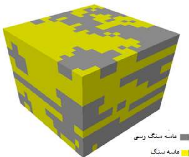
شکل ۱۵: نمونه‌ای از مدل‌های رخساره‌ای حاصل از اعمال روش روند احتمالی لرزه‌ای بر شبیه‌سازی شاخصی متوالی
