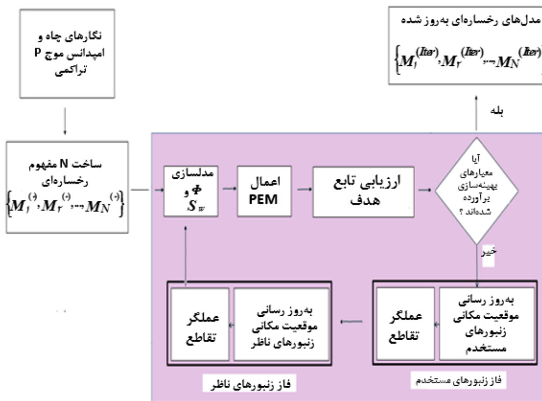
شکل ۷: مراحل اصلی ساخت و به‌روزرسانی مدل‌های رخساره‌ای همخوان با داده‌های نگاره‌ای چاه و امیدانس موج تراکمی بوسیله روش کلونی زنبور مصنوعی - عملگر تقاطع
