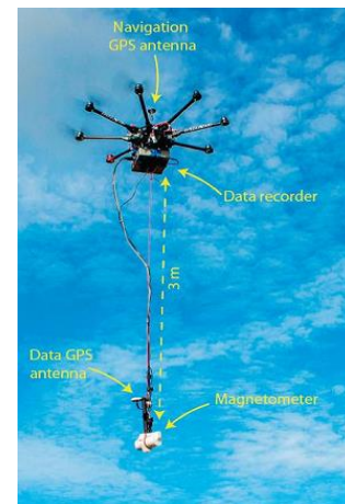
شکل ۸: پهپاد از نوع چند موتوره (Malehmir et al., 2017)
