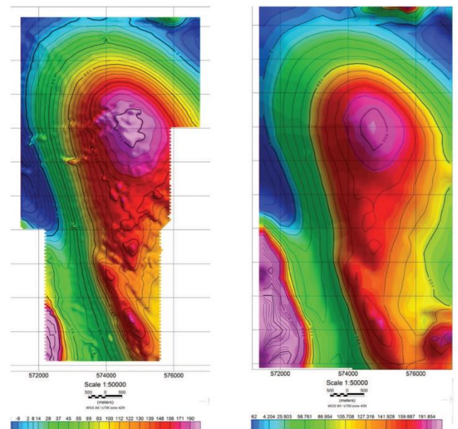
شکل ۱۳. نقشه شدت کل میدان مغناطیسی، سمت راست نقشه به‌دست آمده با استفاده از پهپاد، سمت چپ نقشه به‌دست آمده به روش هوابرد سنتی (Cherkasov and Kapshtan, 2018)
