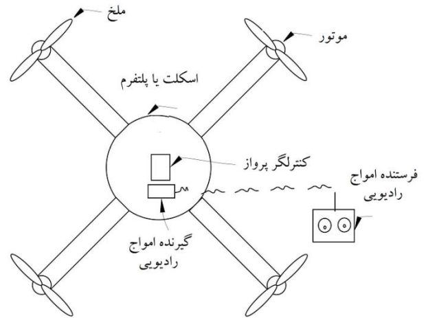
شکل ۶: شماتیکی از مهم ترین اجزای یک پهپاد چهار موتوره
