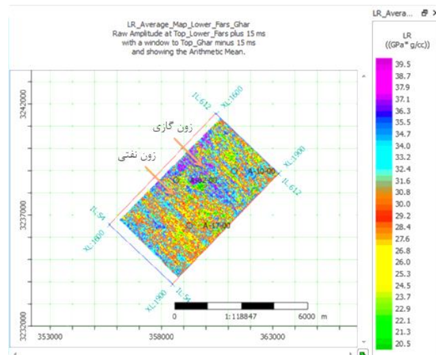
شکل ۱۴: نقشه متوسط \lambda p در بخش کربناته
