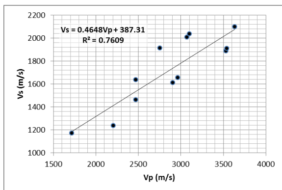
شکل ۹: رابطه‌ی استفاده شده برای ارتباط سرعت امواج برشی و تراکمی
