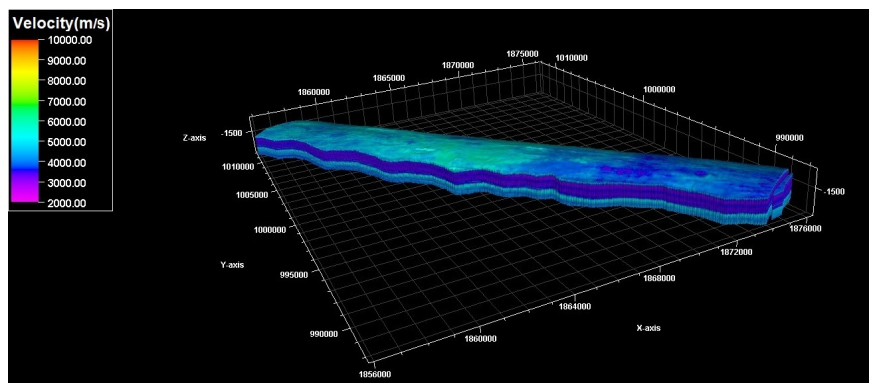
شکل ۵: نمایش سه بعدی از مدل سرعت برای کل مخزن با استفاده از روش شبیه سازی به کمک کوکریجینگ هم مختصات. در این شکل سه بعدی،
