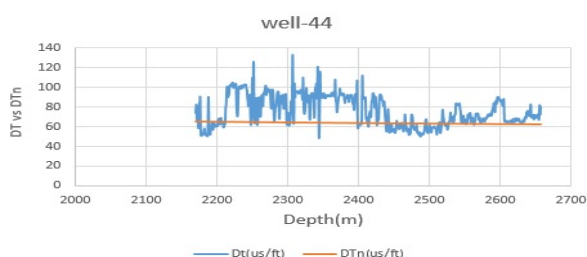
شکل ۱: نمودار صوتی بر روی خط روند طبیعی (قرمز) و نمودار صوتی (آبی) در محل چاه شماره ۴۴.
