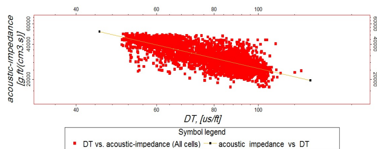
شکل ۳: نمودار تقاطعی داده‌های امپدانس صوتی حاصل از وارون سازی و داده‌های نگار صوتی افزایش مقیاس داده شده در همه زون‌های مخزنی. در این حالت ضریب همبستگی ۷۵ درصد به دست آمد.
