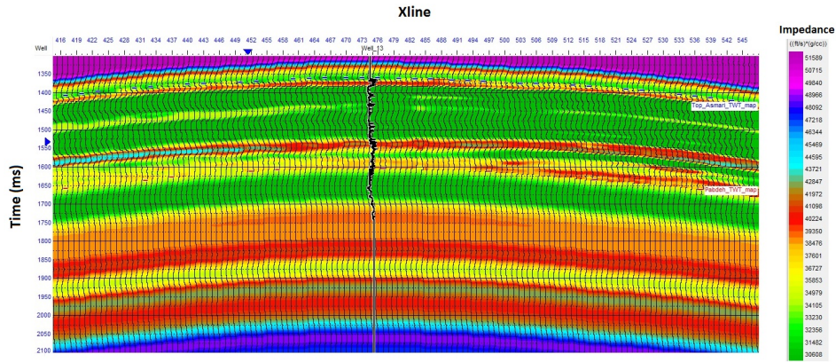
شکل ۲: نمایش مقطع حاصل از وارون سازی لرزه‌ای. در این مقیاس نقشه رنگ امپدانس صوتی (\frac{g}{cm^3}) * (\frac{ft}{s}) است.
