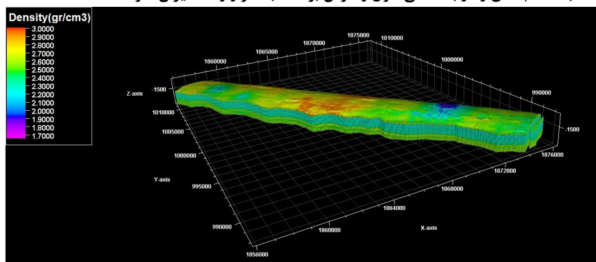
شکل ۶: نمایی سه‌بعدی از مدل چگالی برای کل مخزن با استفاده از روش شبیه‌سازی به کمک کوکریجینگ هم مختصات. در این شکل سه‌بعدی، بعد قائم عمق و دو بعد افقی طول و عرض بر حسب متر و رنگ میزان چگالی (gr/cm³) است.
