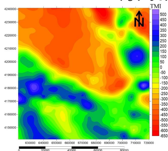
شکل ۶: نقشه شدت میدان مغناطیسی کل پنجره W_6.
