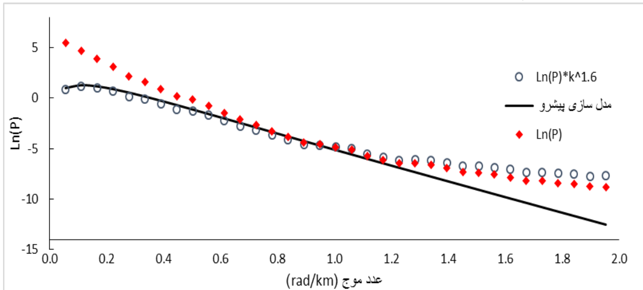
شکل ۹: نتایج بدست آمده با استفاده از روش طیف دی-فرکتال شده. لوزی‌های قرمز طیف توان میانگین شعاعی مشاهده‌ای و دایره‌های آبی طیف دی-فرکتال شده با شاخص فرکتالی ۱/۶ را نشان می‌دهند. خط سیاه مدل برازش شده می‌باشد.
