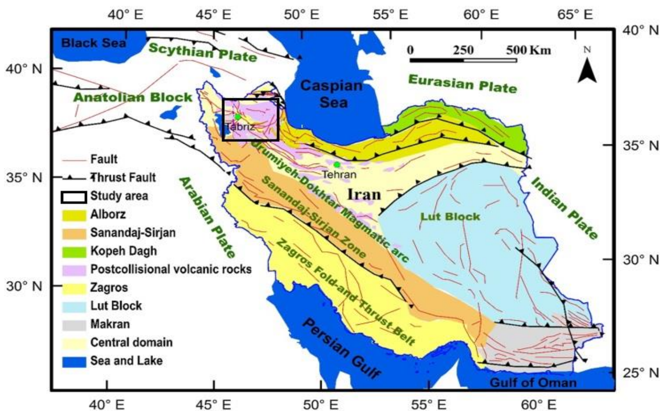
شکل ۲: نقشه زون های ساختاری ایران. مستطیل سیاه رنگ منطقه مورد مطالعه را نشان می دهد (Afshar et al., 2016).
