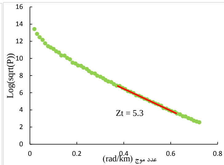
شکل ۷: تخمین عمق بالا با برازش خط راست به دومین بخش از بلندترین قسمت طول موج طیف مشاهده‌ای.
