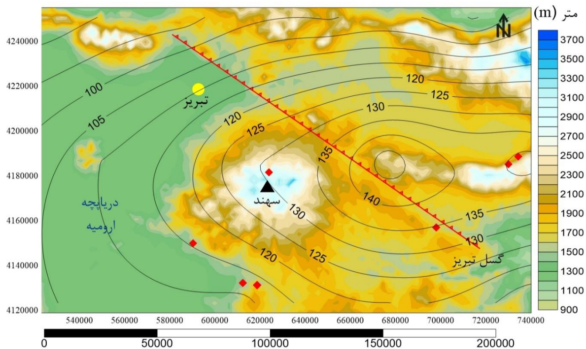
شکل ۱۱: نقشه‌ی تغییرات خطوط تراز جریان حرارتی بر روی نقشه‌ی توپوگرافی شمال غرب ایران تهیه شده از مدل رقومی ارتفاع ۹۰ متر سازمان زمین‌شناسی کشور. قله‌ی سهند در مرکز نقشه و قله‌ی سیلان در قسمت شمال شرق نقشه مشاهده می‌شود (فاصله خطوط کننتوری 5 \text{ mW} / \text{m}^2 می‌باشد).
