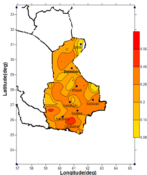
شکل ۳: نقشه پهنه‌بندی شتاب زمین‌لرزه برحسب g در استان سیستان و بلوچستان بر اساس راهکار تعینی.
