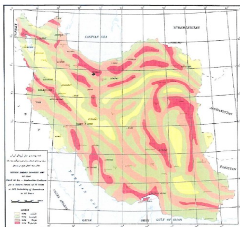
شکل پ-۳: نقشه پهنه‌بندی بیشینه شتاب جنبش زمین برحسب g در ایران برای میانگین دوره بازگشت ۴۷۵ سال (توکل و غفوری آشتیانی، ۱۹۹۹).
