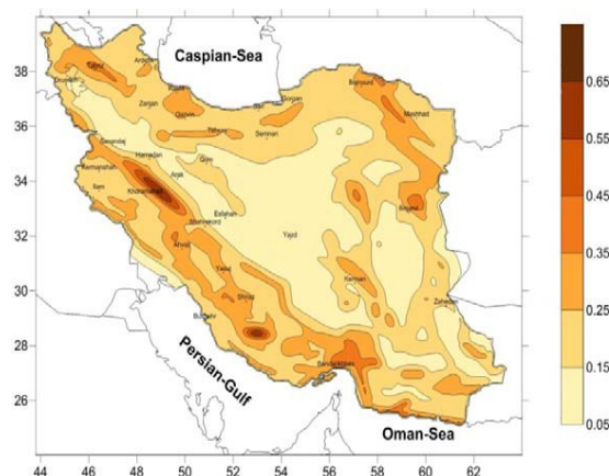
شکل پ-۱: نقشه پهنه‌بندی بیشینه شتاب افقی برحسب g برای ایران برای دوره بازگشت ۴۷۵ سال بر روی سنگ بستر (موسوی و همکاران، ۱۳۹۳).
