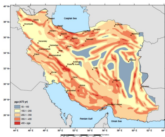
شکل پ-۴: نقشه پهنه‌بندی بیشینه شتاب جنبش زمین برحسب \text{cm/s}^2 در ایران برای میانگین دوره بازگشت ۴۷۵ سال (حمزه‌لو و همکاران، ۲۰۱۲).
