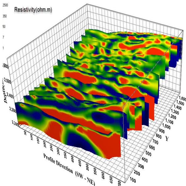
شکل ۲۰: نمایش ۲/۵ بعدی مقاطع مقاومت ویژه با استفاده از نرم‌افزار ZondRes2D.
