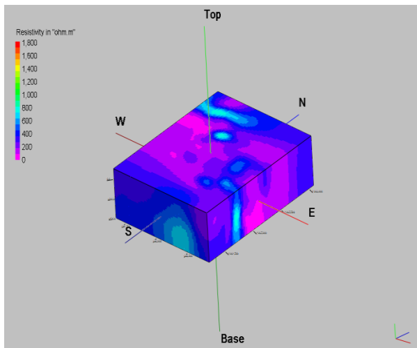
شکل ۳۳: نمایش سه بعدی داده‌های مقاومت ویژه توسط نرم افزار
