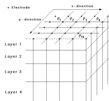
شکل ۱۷: مدل سه‌بعدی زیر سطح زمین که توسط نرم‌افزار Res3dinv به تعدادی لایه و بلوک‌های مکعبی شکل با مقادیر مقاومت ویژه متفاوت تقسیم می‌شود (Loke, 2002).
