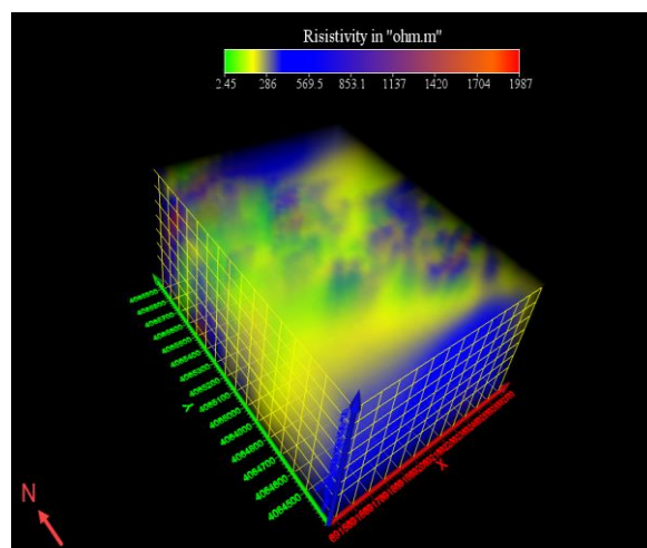
شکل ۳۱: نمایش سه بعدی داده‌های مقاومت ویژه توسط نرم افزار
