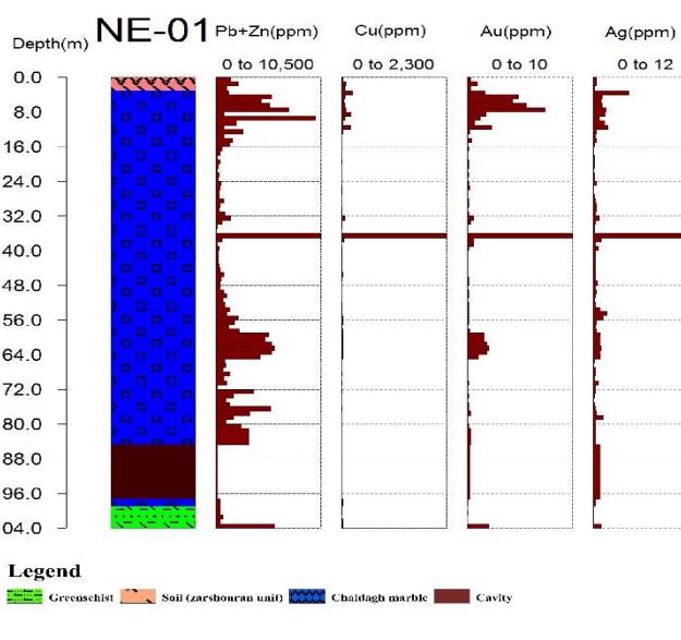
شکل ۳۶: نمودار ترسیم‌شده گمانه NE_01.
