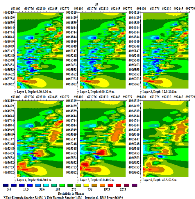
شکل ۲۴: مقاطع افقی حاصل از مدل سازی سه بعدی مقاومت ویژه (از سطح تا عمق ۵۲/۵ متر).
