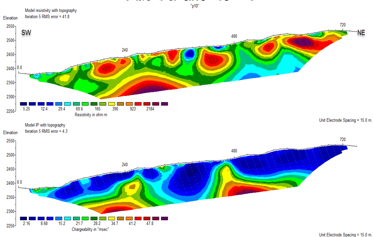
شکل ۱۹: نتایج و مقاطع وارون سازی دوبعدی پروفیل ۱۰.
