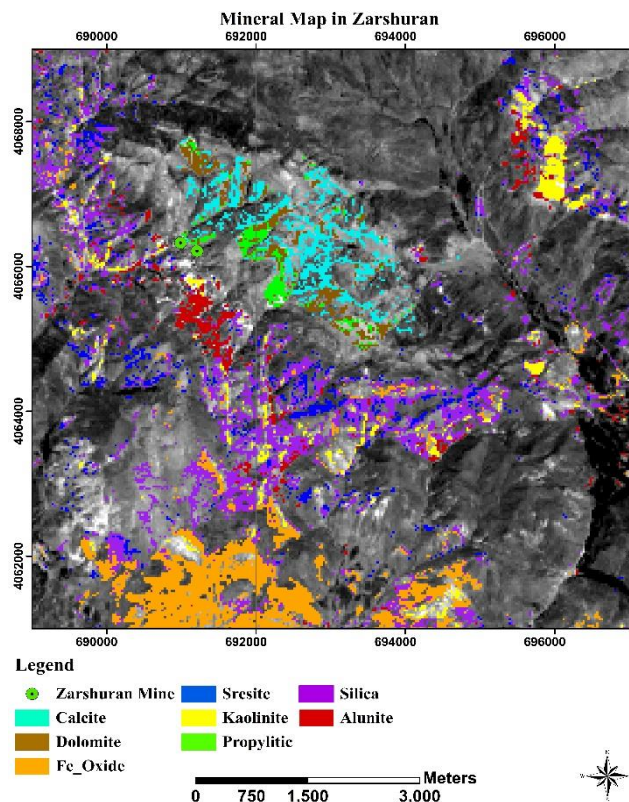
شکل ۱۴: نقشه نگاشت کانی‌های استخراج‌شده از تصویر ASTER با استفاده از روش SAM.
