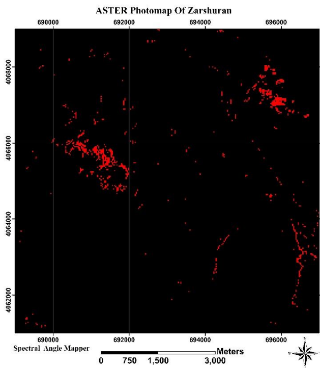
شکل ۱۳: تصویر حاصل از روش SAM (پیکسل‌های قرمز مناطق دگرسانی آرژلیک را نشان می‌دهند).
