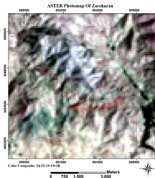
شکل ۷: مناطق دگرسانی سیلیسی به رنگ قرمز در تصویر حاصل از باندهای TIR, 10, 12, 14.
