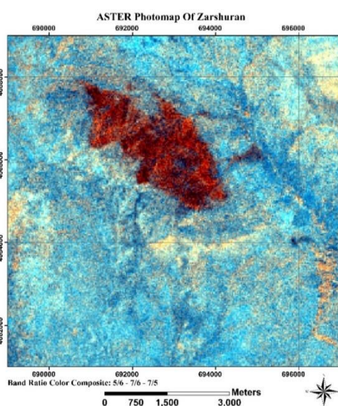
شکل ۵: ترکیب رنگی نسبت باندی RGB:5/6-7/6-7/5 سنجنده ASTER که در آن مناطق دگرسانی آرژیلیک و آرژیلیک پیشرفته به رنگ زرد مایل به خاکستری دیده می شود.
