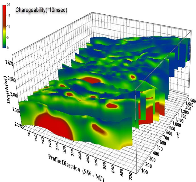
شکل ۲۱: نمایش ۲/۵ بعدی مقاطع قطبش‌القایی با استفاده از نرم‌افزار ZondRes2D.
