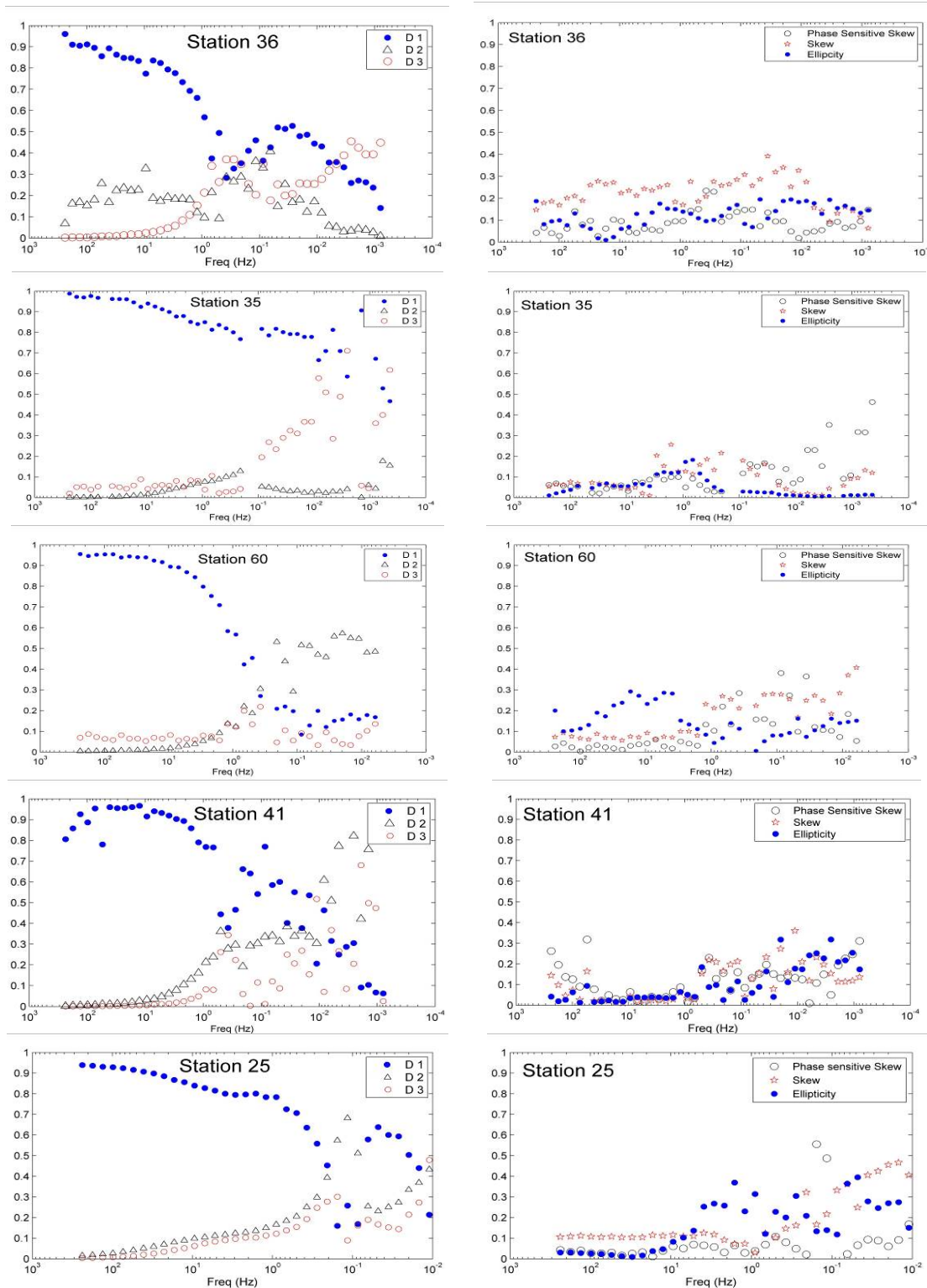
شکل ۷: مقادیر چولگی، بیضی‌وارگی، چولگی حساس به فاز و اندیس‌های وزنی نرمال برای ایستگاه‌های ۳۵، ۳۶، ۴۱ و ۲۵.
