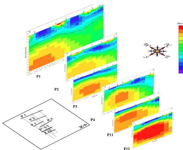
شکل ۱۲: نمایش موازی مقاطع شمالی - جنوبی مقاومت ویژه حاصل از مدل‌سازی دوبعدی وارون داده‌های دو مد TE و TM.
