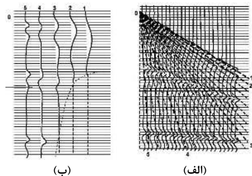
شکل ۱: تصویر شماتیک از تبدیل ردلرزه شعاعی. الف) رکورد چشمه مشترک لرزه‌ای (ب) ردلرزه شعاعی استخراج شده از حوزه x-t با استفاده از مجموعه‌ای از دامنه‌های لرزه‌ای در امتداد یک مسیر خطی با سرعت یا زاویه ثابت (هنلی، ۲۰۰۳).
