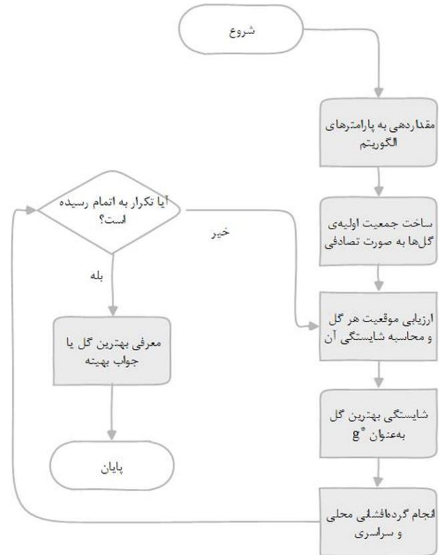
شکل ۲: فلوجارت الگوریتم گردهافشانی گل.
