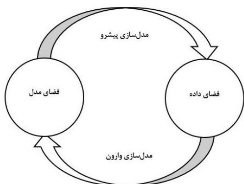
شکل ۱: ارتباط بین فضای مدل و داده‌های مرتبط با آنها در یک مساله پیشرو و وارون (Roy, 2007).
