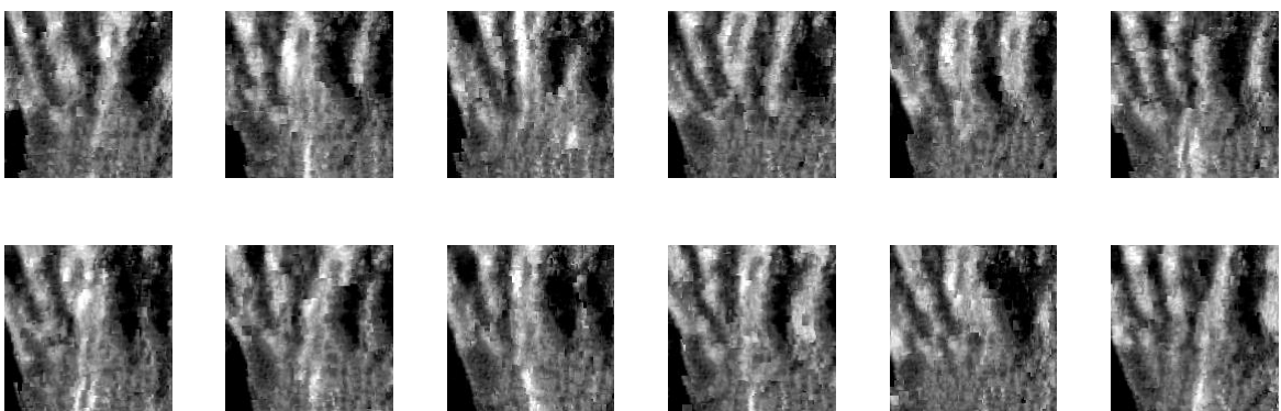
شکل ۳: چند تحقیق تولید شده با روش زمین آمار چند نقطه ای DisPat بر اساس تصویر آموزشی سیستم دلتایی ناپایستا
