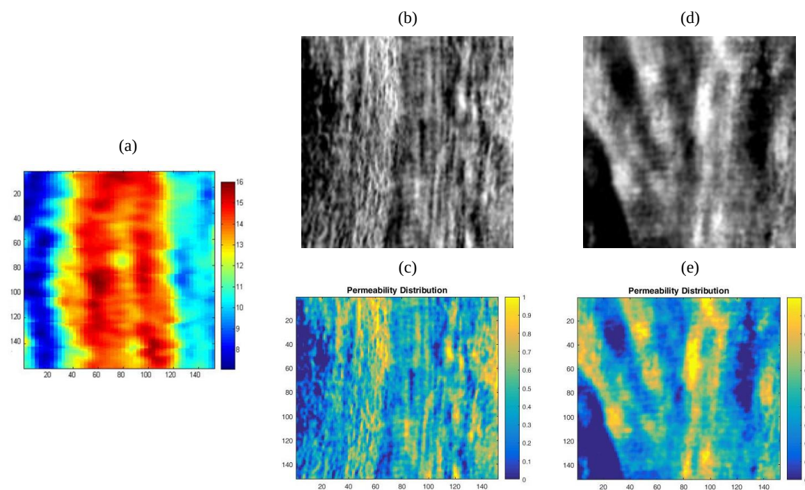
شکل ۱: (a) توزیع تخلخل برای مدل شبیه‌سازی مخزن؛ (b) تصویر آموزشی شبکه شکستگی ایستا؛ (c) توزیع تراوایی متناظر با (a) ورودی به مدل شبیه‌سازی مخزن؛ (d) تصویر آموزشی دلتای نایستا؛ (e) توزیع تراوایی متناظر با (d) ورودی به مدل شبیه‌سازی مخزن بر این اساس، روش‌های زمین آمار چند نقطه ای برای ایجاد تعداد زیادی از مدل های تصادفی بکار گرفته شدند. تعداد اندکی از تحقیقات
