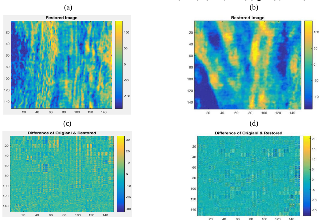
شکل ۵: (a) مدل تراوایی فشرده تنک برای شبکه شکستگی با استفاده از لغت نامه آموزش یافته با روش ILS-DLA و (b) همان، برای سیستم دلتایی؛ (c) تفاوت بین مدل اصلی و مدل فشرده برای سیستم شکستگی؛ (d) همان، برای سیستم دلتایی
