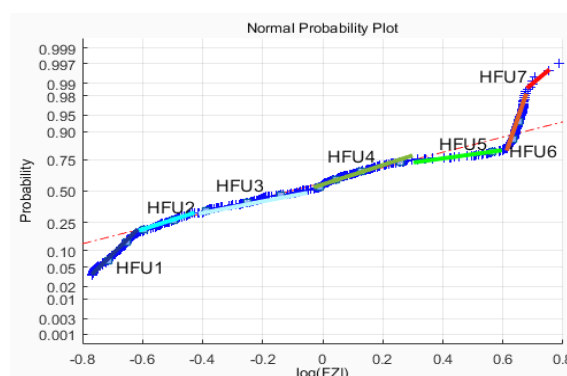
شکل ۱: نمودار احتمال لگاریتم شاخص زون جریان در چاه W-1.
