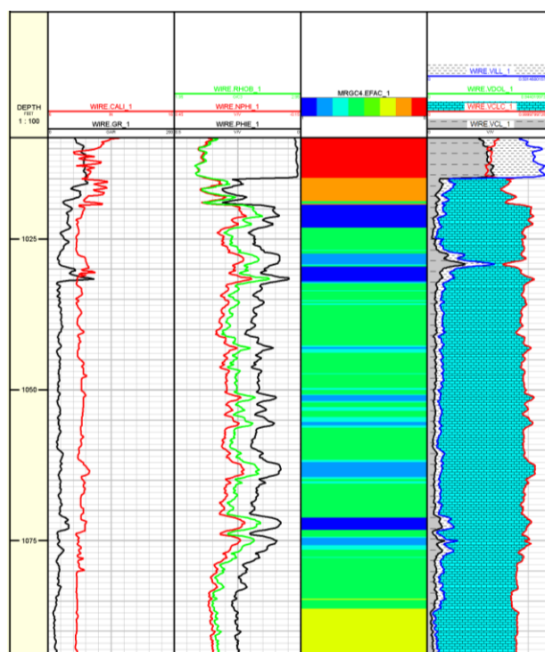
شکل ۱۱: نمایش رخساره‌های الکتریکی حاصل از روش MRGC در چاه W-1.
