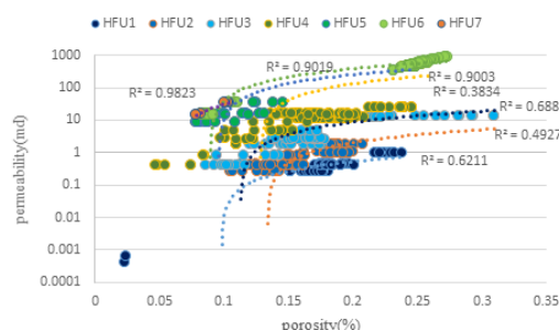
شکل ۴: نمودار توزیع تخلخل - تراوایی برای هر یک از واحدهای جریان مربوط به مخزن مورد مطالعه در چاه W-1.
